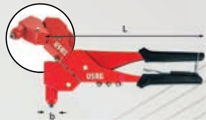
U09950006 Klešta jednoručna za pop nitne 2,4-4,8 mm
