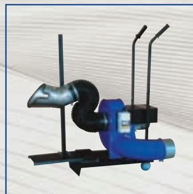
Mobilni uređaj za odsisavanje vazduha, lako podesiv za sve tipove putničkih vozila.
